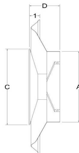
CORTE X-X
