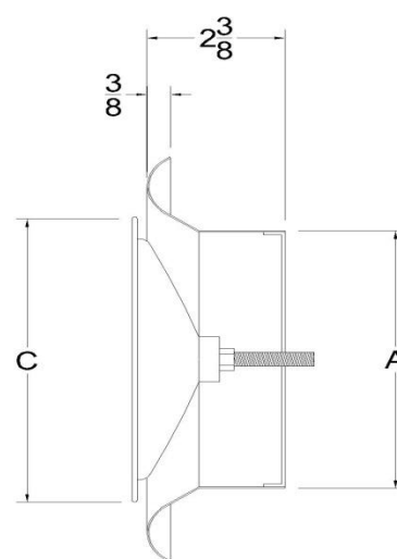
CORTE X-X
